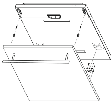
Рис. 4 Установка внешней панели
